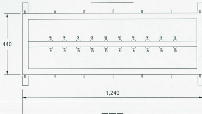
正面図
