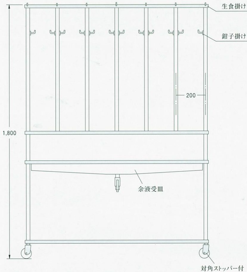
正面図
